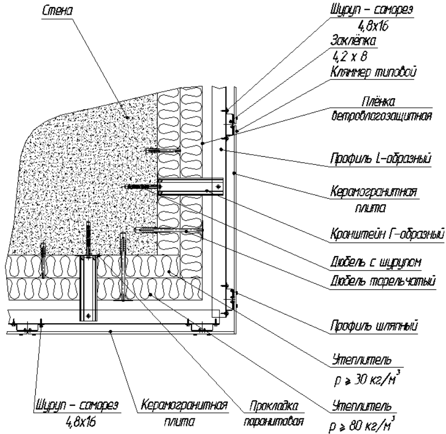
Узел 3. Угол наружный - разрез горизонтальный
