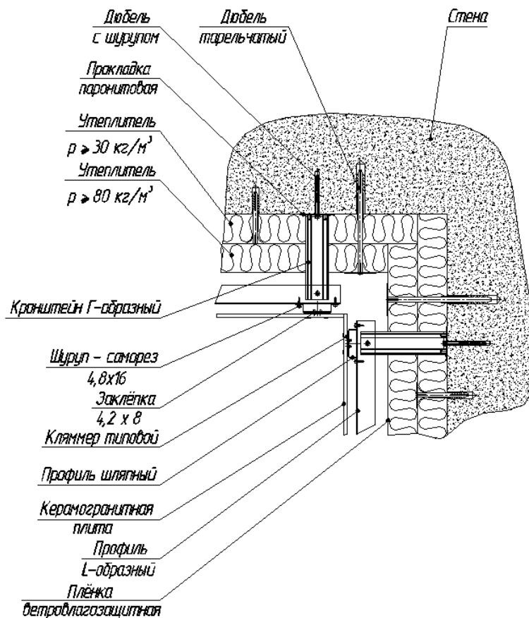
Узел 4. Угол внутренний - разрез горизонтальный
