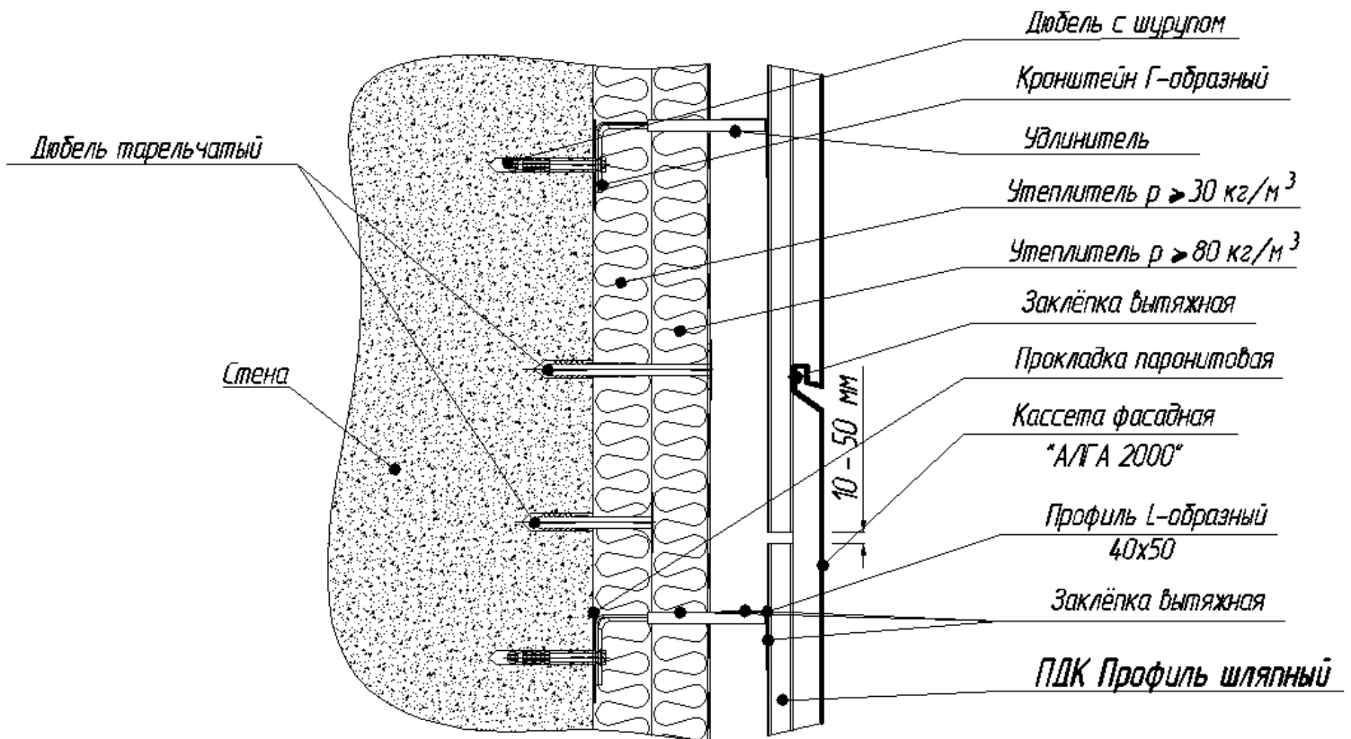
Узел 1. Шов горизонтальный - разрез вертикальный
