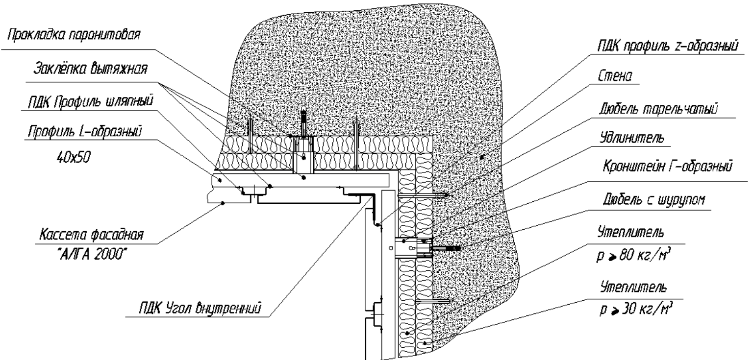
Узел 4. Угол внутренний - разрез горизонтальный
