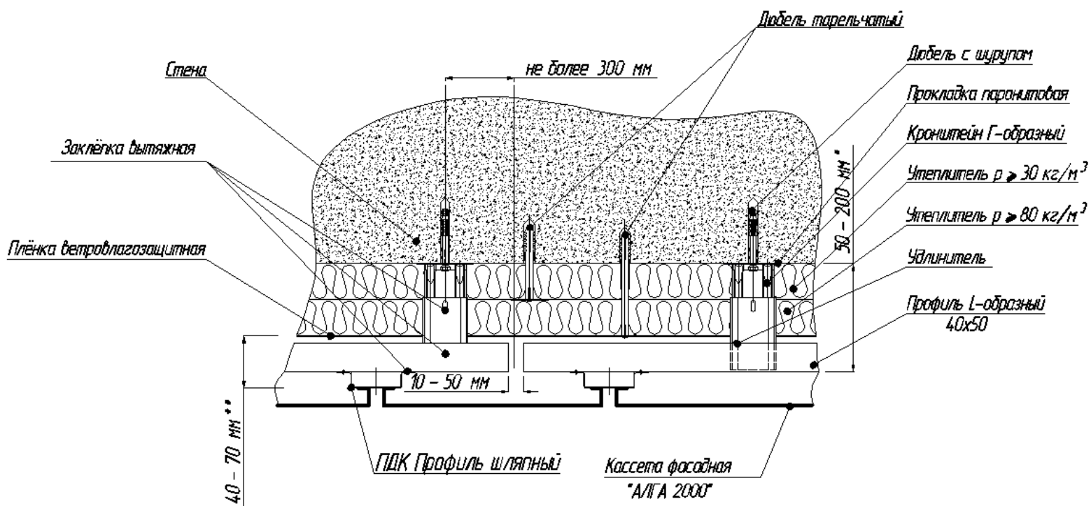
Узел 1. Шов горизонтальный - разрез вертикальный
