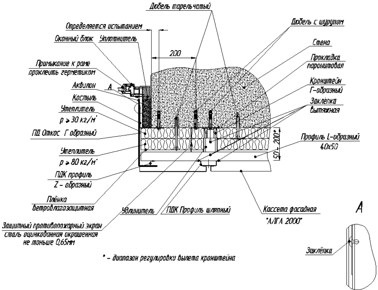
Узел 6. Боковой откос окна - разрез горизонтальный
